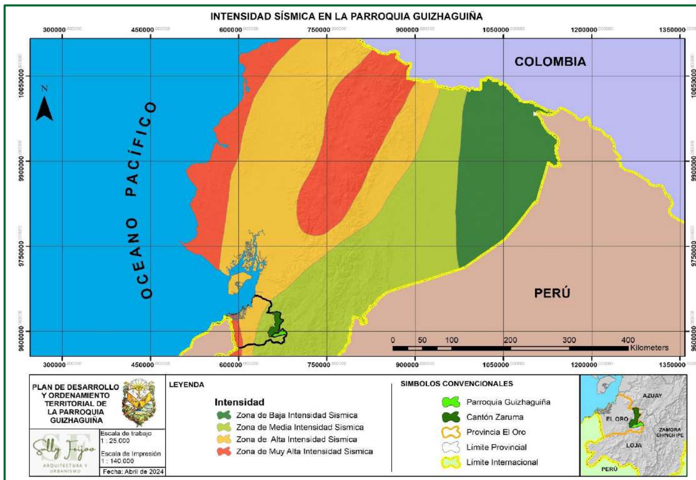
Mapa FA 22: Intensidad Sísmica en la parroquia Guizhagüiña
