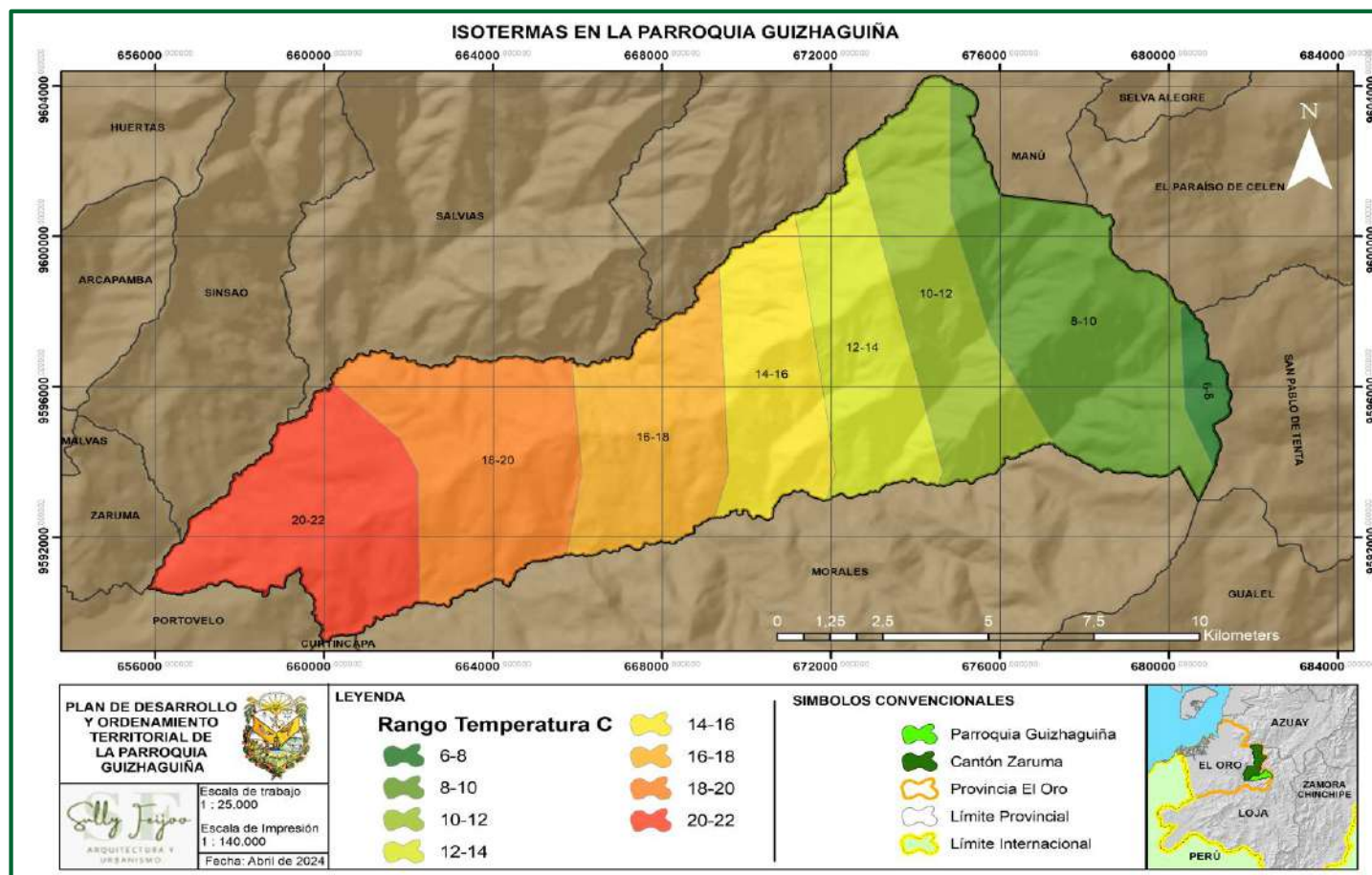
Mapa FA 27: Isotermas de la parroquia Guizhagüiña
