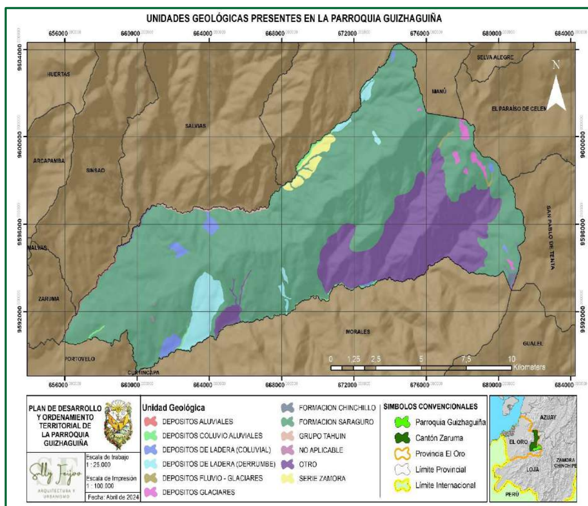
Mapa FA 9: Unidades Geológicas presentes en la parroquia Guizhagüña
