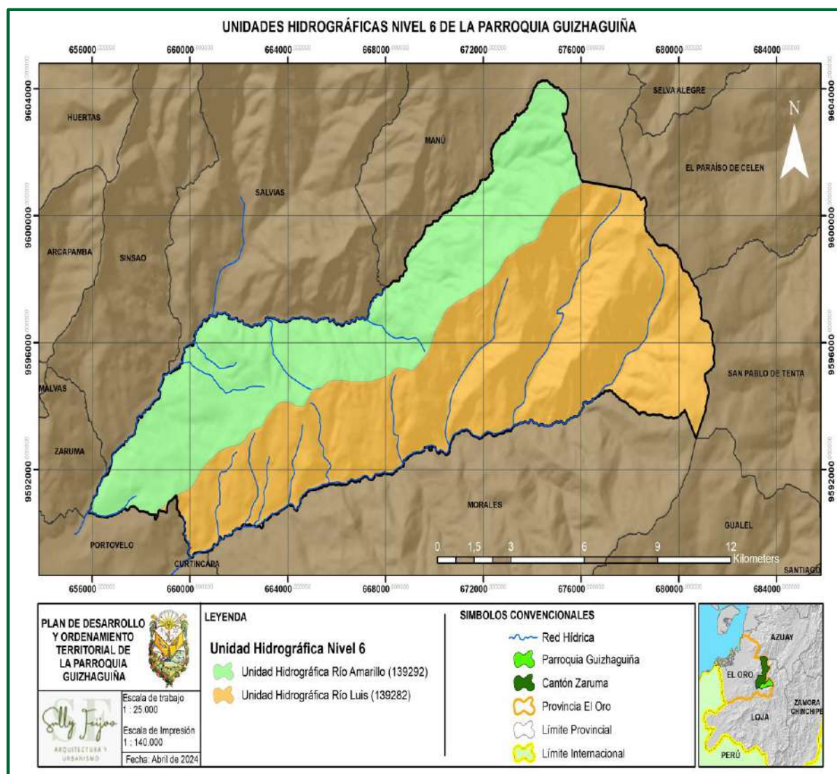
Mapa FA 2: Unidades Hidrográficas Nivel 6 de la parroquia Güizhagüiña
