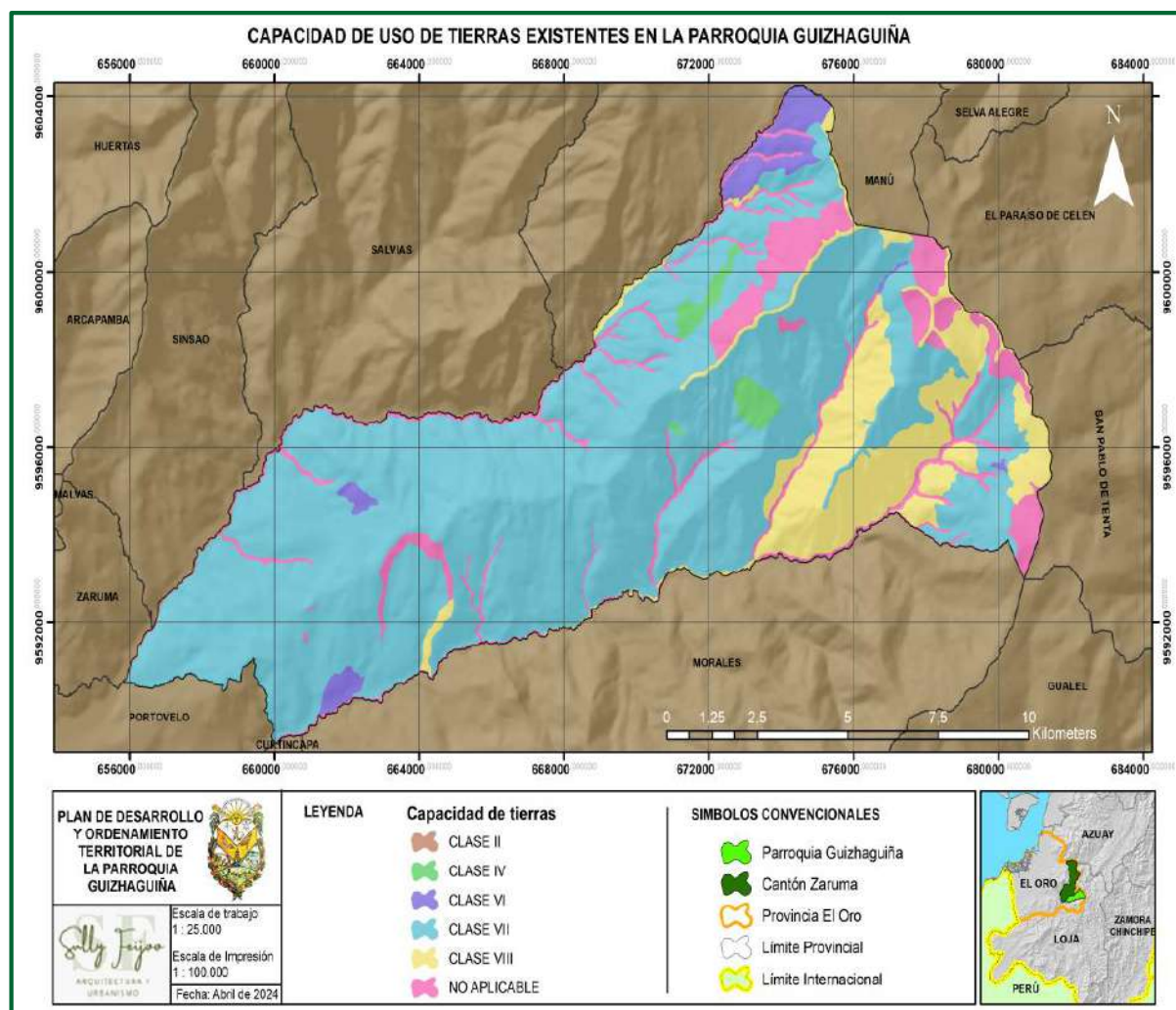
Mapa FA 12: Capacidad de uso de tierras presentes en la parroquia Güizhagüña
